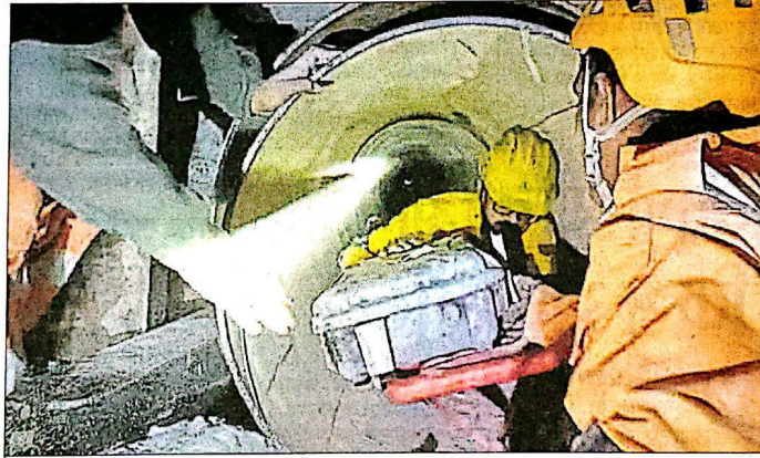
सिलक्यारा सुरंग में शुक्रवार को 800 एमएम पाइप के भीतर जाकर मलबे की जाँच कर उपकरणों के साथ लौटते एक्सपर्ट। इसी उपकरण से पता किया गया कि मलबे में आगे का 5.4 मीटर का रास्ता साफ है। • हिन्दुस्तान
